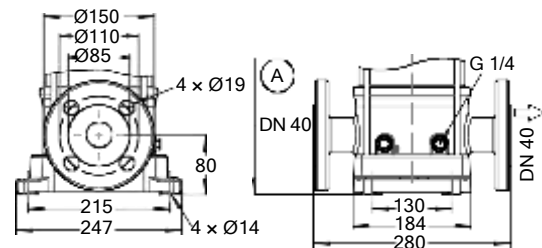
Fig. 25: Movitec VF, VSF
