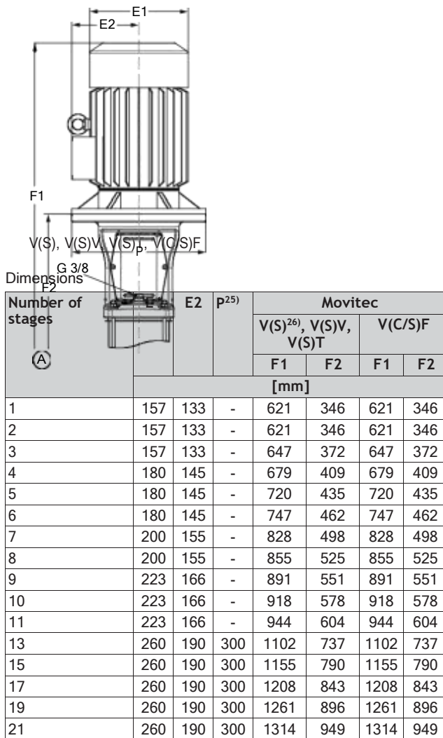
Fig. 28: Movitec VV, VSV
