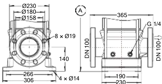
Fig. 56: Movitec VF/VSF; PN 16
