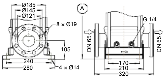
Fig. 43: Movitec VCF
