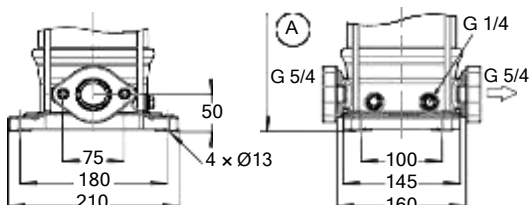
Fig. 16: Movitec V/VS
