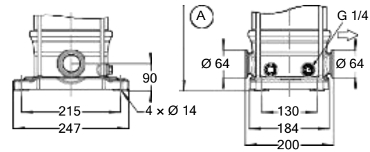
Fig. 39: Movitec VT, VST
