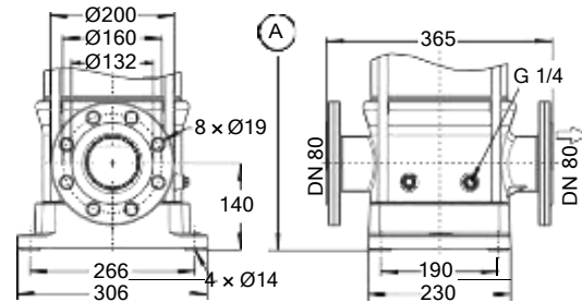
Fig. 49: Movitec VF, VSF; PN 16, 25
