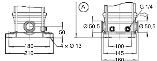
Fig. 6: Movitec VT, VST
