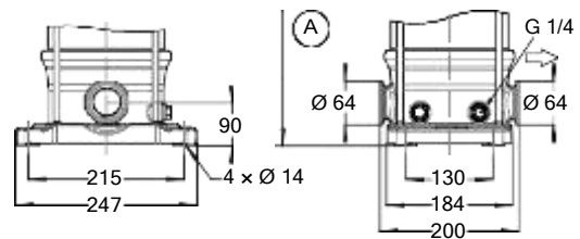
Fig. 34: Movitec VT, VST
