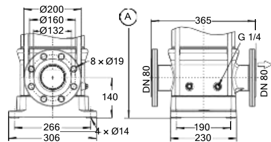
Fig. 46: Movitec VF, VSF
