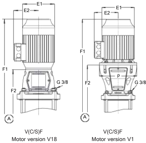
Fig. 48: Movitec VCF
