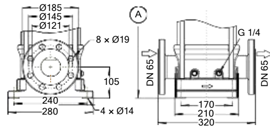
Fig. 45: Movitec VCF
