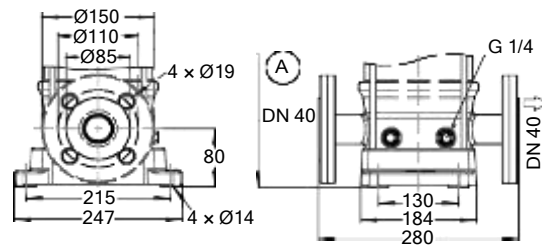
Fig. 26: Movitec VCF
