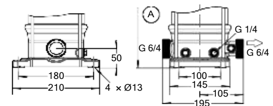
Fig. 21: Movitec VME
