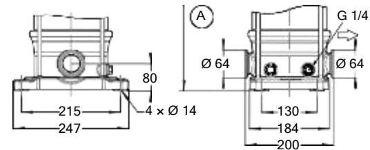
Fig. 29: Movitec VT, VST
