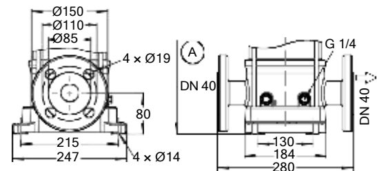
Fig. 30: Movitec VF, VSF
