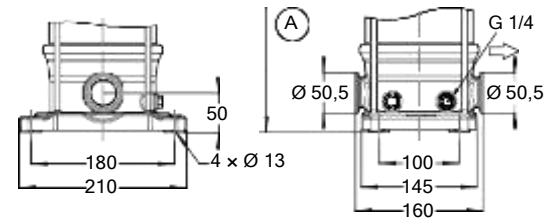
Fig. 18: Movitec VT/VST
