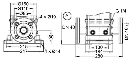
Fig. 31: Movitec VCF
