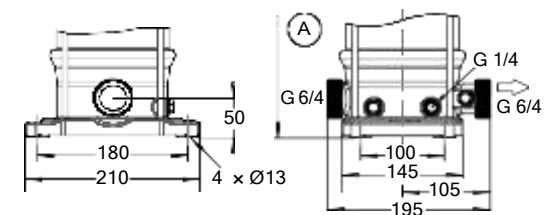
Fig. 9: Movitec VME
