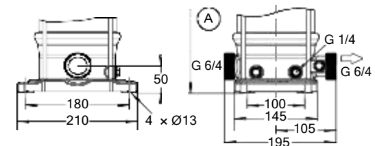
Fig. 15: Movitec VME
